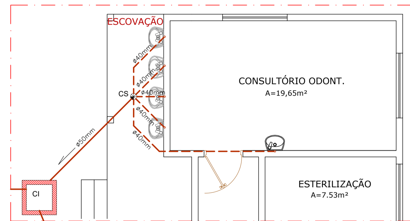
DETALHE INST. SANITÁRIA - ESCOVAÇÃO E LAVATÓRIO DO CONS. ODONT. - ESC.:1/50
