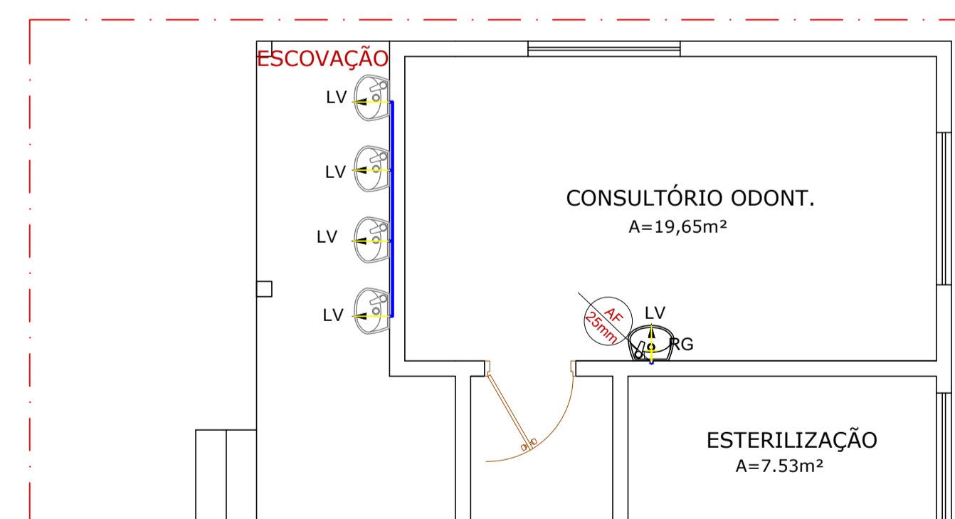
DETALHE INST. HIDRÁULICA - ESCOVAÇÃO E LAVATÓRIO DO CONS. ODONT. - ESC.:1/50
