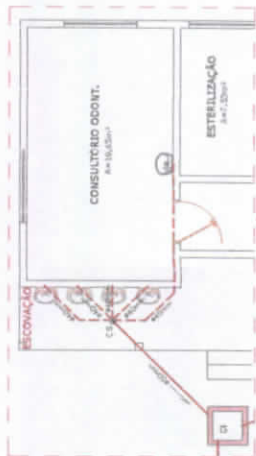
DETALHE INST. SANITÁRIA - ESCOVAÇÃO E LAVATÓRIO DO CONS. ODONT. - ESC. -1/50
