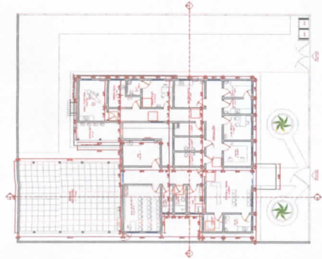
NÍVEL 01 - NÍVEL DO TERRENO ESC. 1/200
